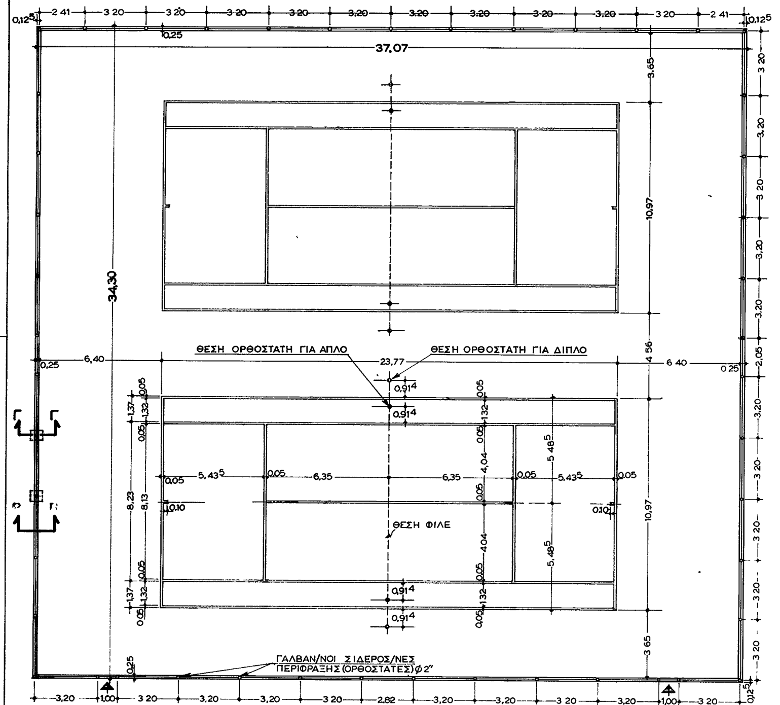
ΚΑΤΩΗ ΓΗΠΕΔΩΝ ΚΛ. 1:200
