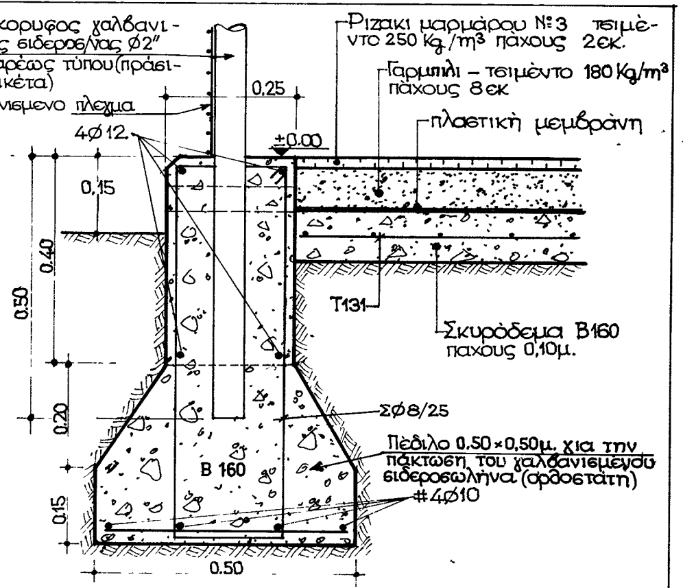
ΤΟΜΗ Γ-Γ ΚΛ. 1:10 ΚΑΤΑΣΚΕΥΗ ΓΗΠΕΔΟΥ ΜΕ ΥΛΙΚΟ ΤΥΠΟΥ ΚΟΥΚΙ
