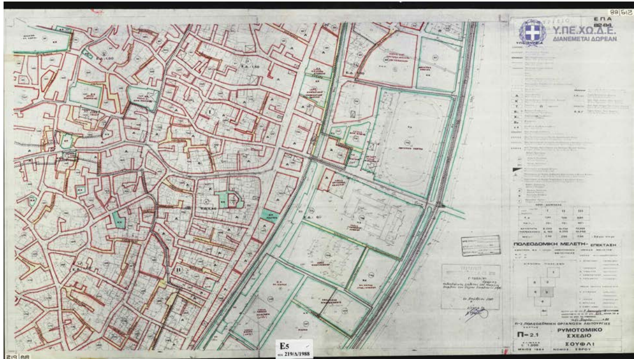
Χάρτης 11. Ρυμοτομικό Σχέδιο Σουφλίου (ΦΕΚ 219/Δ'/11-03-1988, Π.Δ. 07-01-1988)
